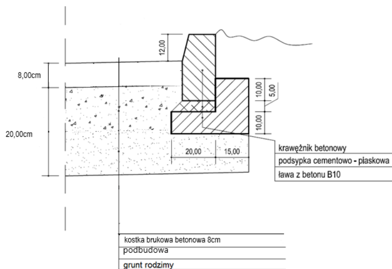
Rys.2. Szczegół konstrukcji
