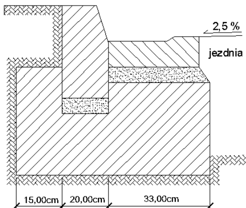
Rys.1. Przekrój pionowy poprzeczny
